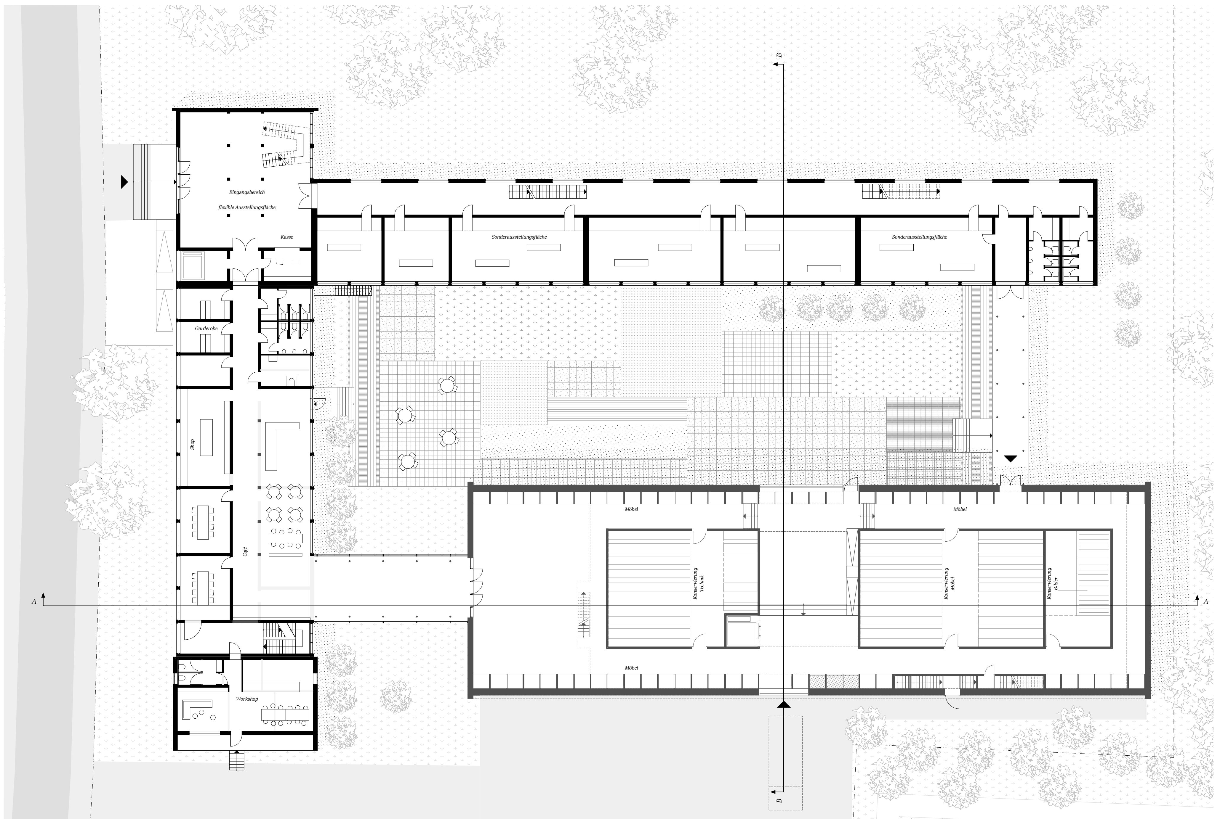
Erdgeschoss 1:200
