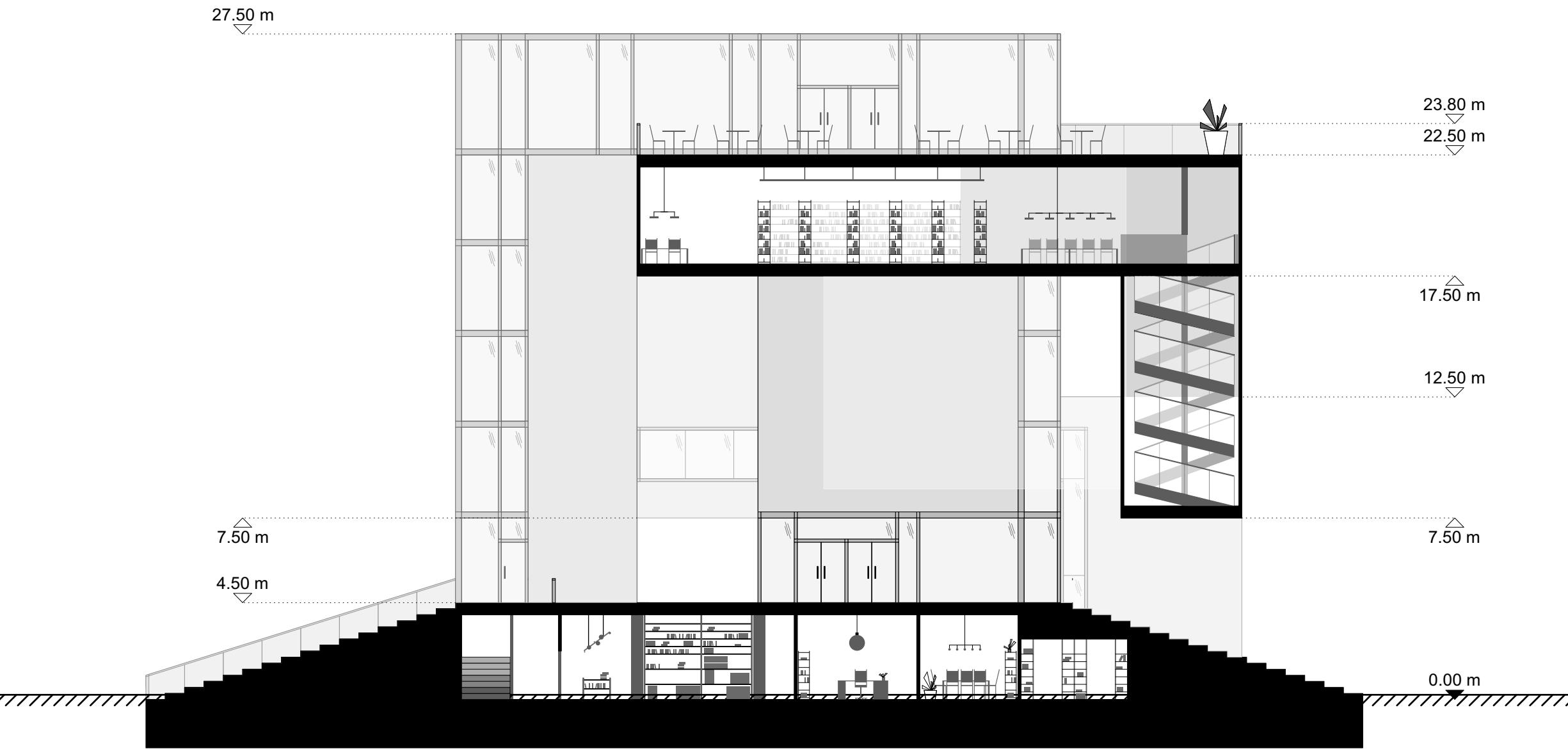
Schnitt A 1:200
