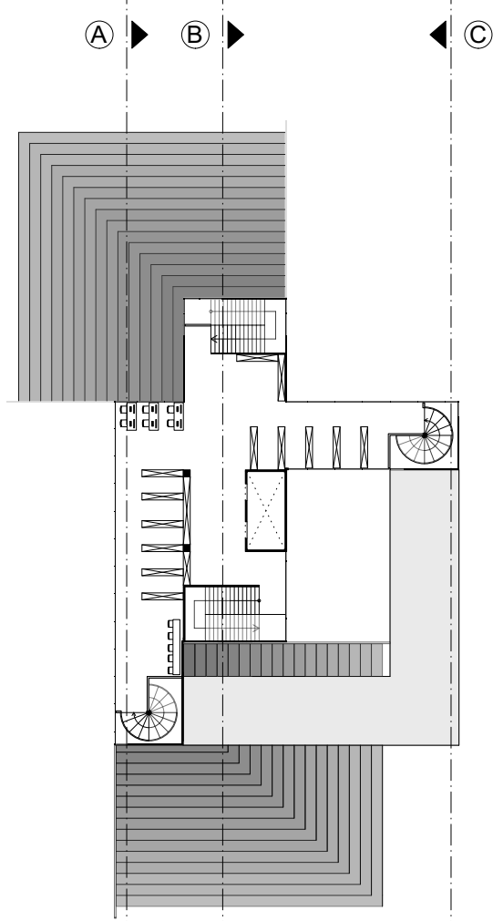
Schnitt bei 19 m
