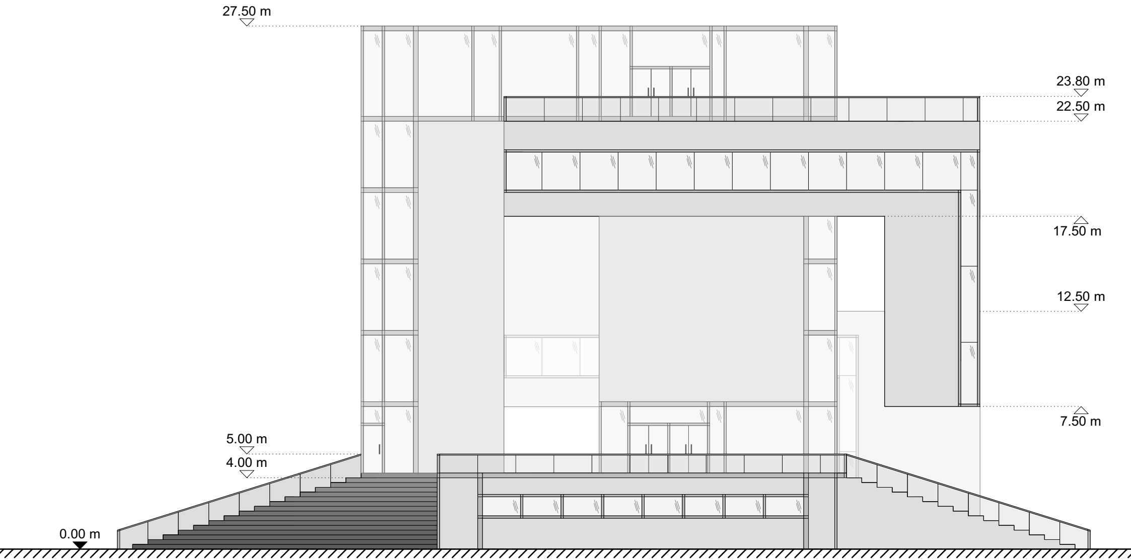
Ansicht West
