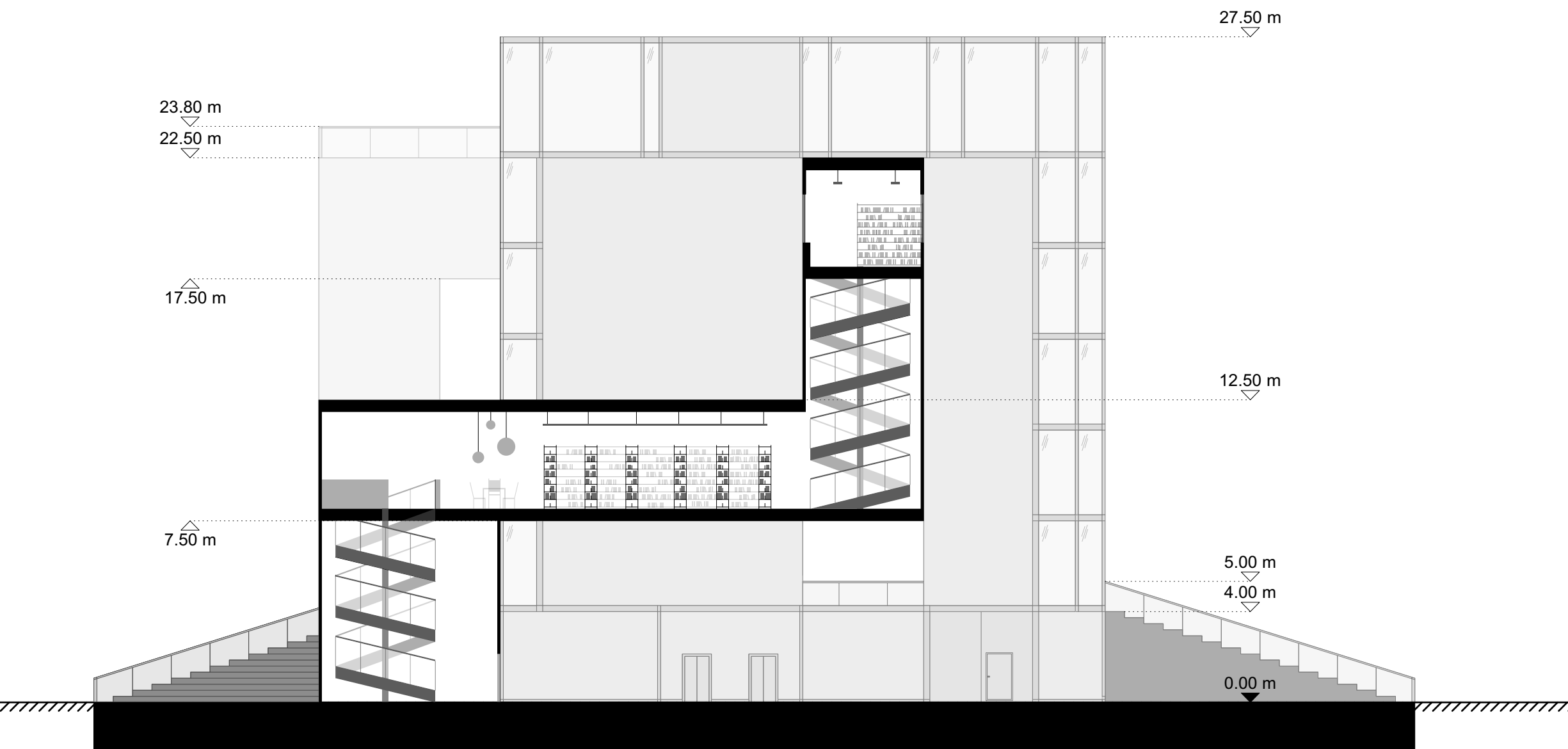
Schnitt C 1:200
