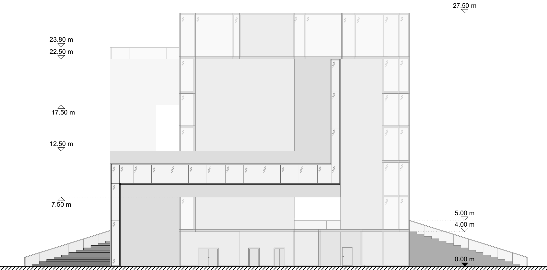
Ansicht Ost
