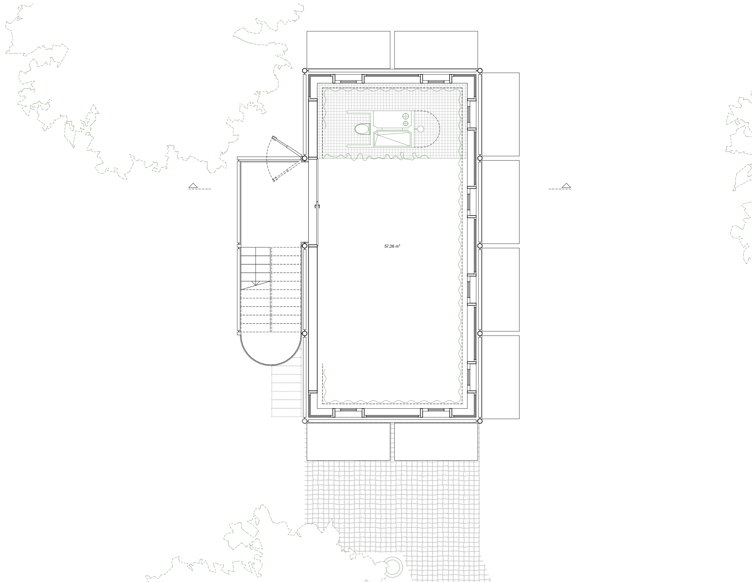
Grundriss Zoom-In, Grundriss 1. Obergeschoss Leipzig Mockau, Walter-Albrecht-Weg
