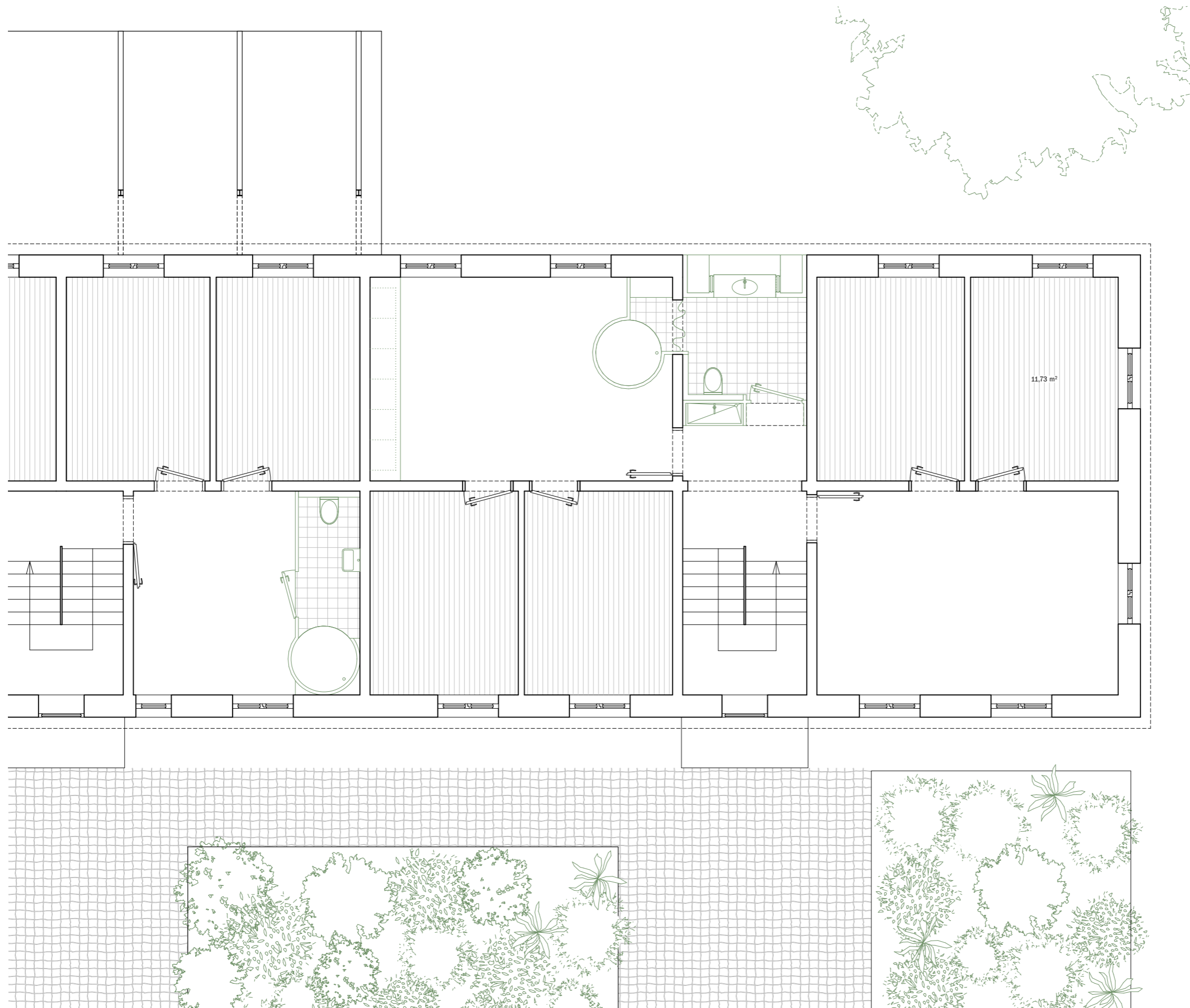
Grundriss Zoom-In, 1. Obergeschoss Leipzig Mockau, Walter-Albrecht-Weg
