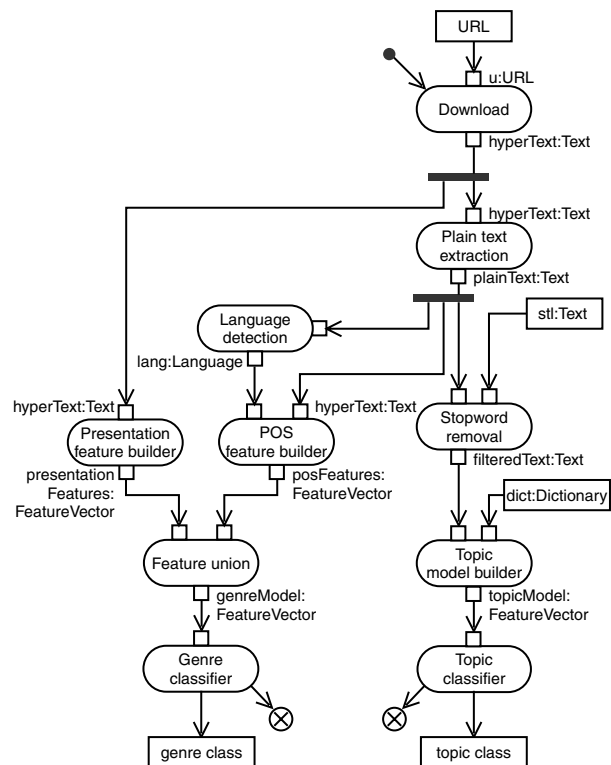
Abbildung 5: IR-Prozess für die Kategorisierungsaufgabe, spezifiziert als UML Aktivitätsdiagramm.
