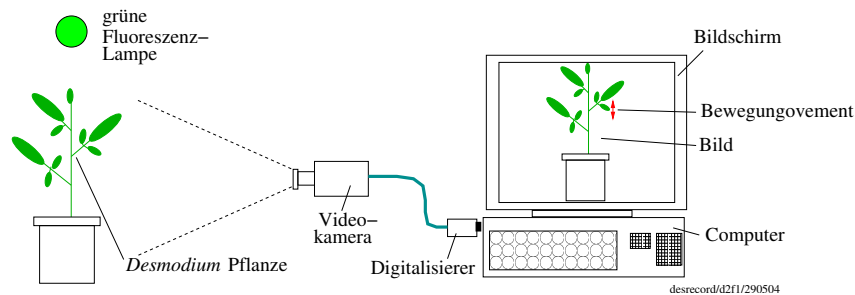
Abbildung 2.1.: Registrierung der Blattbewegung mit einem Bildanalysator über einen Computer. Das sich bewegende Objekt wird über eine Videokamera aufgenommen, im Framegrabber digitalisiert und über den Computer auf den Bildschirm übertragen. Die Daten werden zur weiteren Analyse gespeichert.
