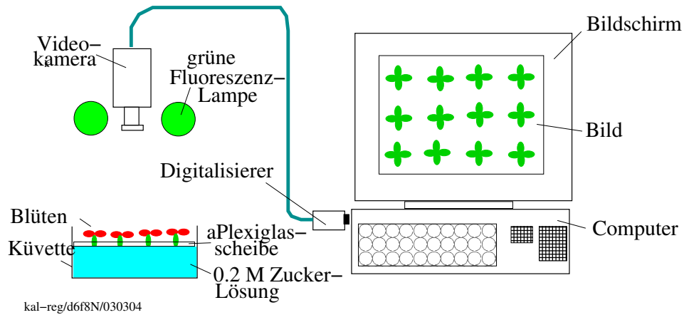
Abbildung 6.8.: Küvette mit Kalanchoe -Blüten. Polyurethanscheibe mit Löchern für die Blütenstiele, Zuckerlösung in dem Plastikgefäß. Beleuchtung mit zwei grünen Leuchtstoffröhren, zusätzlich mit grüner Folie umwickelt. Registrierung mit Video-Kamera und Digitalisierung des Bildes über einen Framegrabber und Computer. Die Blüten werden auf dem Monitor gezeigt.
