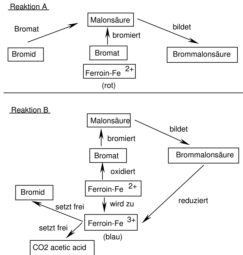
Abbildung 5.2.: Reaktionsschema der Belousov-Zhabotinsky-Reaktion mit den beiden Teilreaktionen A und B.
