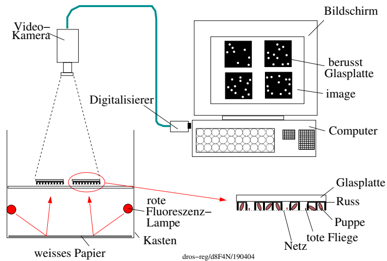
Abbildung 8.8.: Registrieranlage zum Messen des Schlüpfens von Drosophila -Fliegen aus dem Puparium mit Video-Kamera, Digitalisierer und Computer mit Hilfe der Russ-Methode. Licht von zwei roten Leuchtstoffröhren wird von einem weissen Papier auf die Unterseite von Puppenhaltern reflektiert, von denen eine im unteren rechten Teil der Abbildung genauer gezeigt ist: Eine Metallplatte mit 10*10 Löchern, jedes mit einer Puppe. Ein weisses feinmaschiges Netz verhindert, daß die Puppen herausfallen. Geschlüpfte Fliegen wischen den Russ auf der Unterseite der Glasplatten ab. Rotes Licht kann an diesen Stellen von der kamera gesehen werden (siehe Bildschirm und Abbildung 8.9). Die Daten werden gespeichert und als Funktion der Zeit aufgetragen (siehe Abbildung 8.10).
