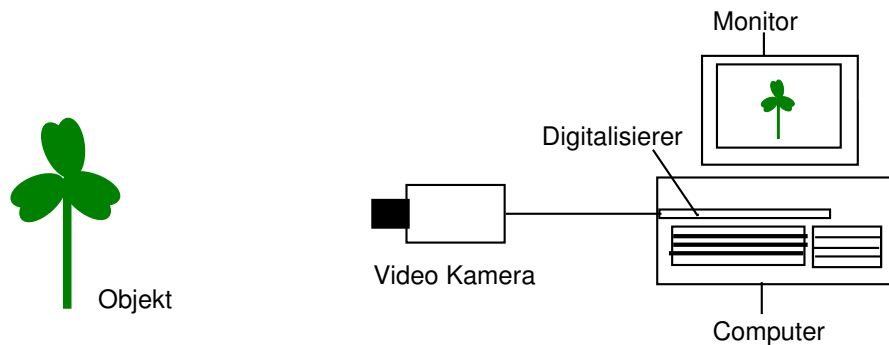
Abbildung 6.4.: Registrierung der Oxalis -Blattbewegung mit Video-Digitalisierung und Computer
