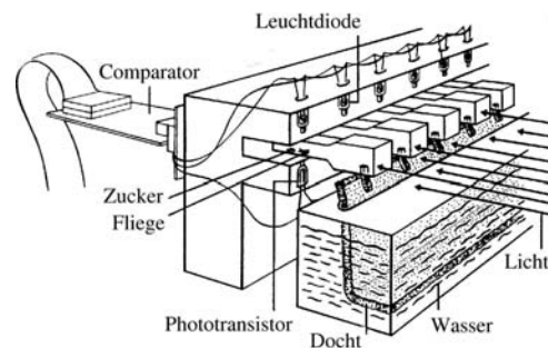
Abbildung 8.6.: Registrieren der Aktivität von Drosophila in Küvette mit Infrarot-Lichtschranke und Computersystem.
