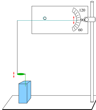
Abbildung 1.7.: Registrieren der Seitenfiederbewegung von Desmodium motorium nach Koukkari et al. (1987). An der Spitze des Seitenfiederblättchens ist ein feiner Faden oder ein Haar mit etwas (!) wasserlöslichem Klebstoff befestigt, der an einer feinen Drahtwippe hängt. Der Zeiger der Wippe gibt den Winkel des Blättchens an.
