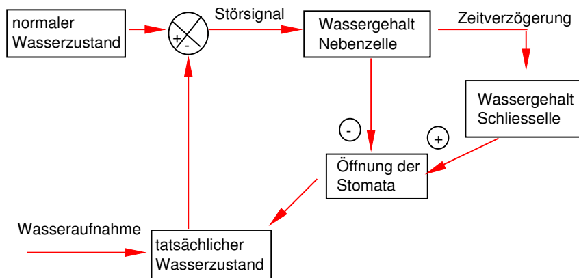
Abbildung 5.8.: Wie Transpirationsschwingungen bei einem Haferblatt entstehen: Schema des Rückkopplungskreises. Der augenblickliche Zustand der Wasserversorgung wird mit dem Sollwert verglichen (im oberen Kreis mit + und - Zeichen). Falls ein Unterschied existiert, wird dieser als Fehlersignal benutzt, um die Stomataweite zu beeinflussen (schliessen der Stomata, wenn der Wasserzustand zu niedrig ist, öffnen, wenn er zu hoch ist). Zeitverzögerungen sind für das Auftreten von Schwingungen wichtig.
