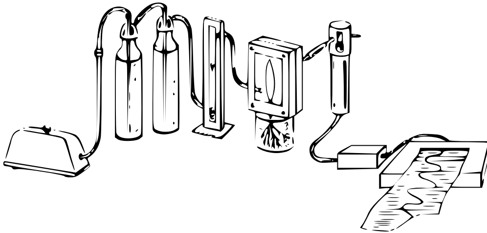
Abbildung 5.9.: Haferkeimling mit Primärblatt in Küvette, um die Transpiration zu messen. Unter der Küvette ein Gefäß mit Wasser für die Wurzeln. Die Aquariumpumpe drückt Luft durch die beiden Waschflaschen mit trockenem Silikagel. Die trockene Luft gelangt in die Küvette und wird vom Haferblatt durch Transpiration angefeuchtet. Die Feuchte wird elektronisch gemessen, das Signal verstärkt und über einen Spannungsschreiber registriert. }
