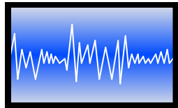
EEG
