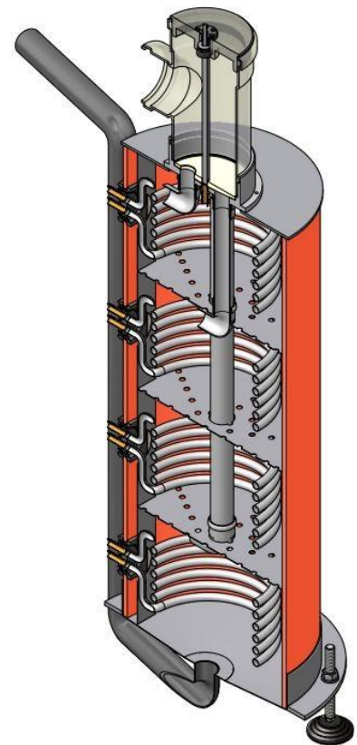
Abb. 1: Schematische Verfahrensdarstellung (Foto: Revincus GmbH)
