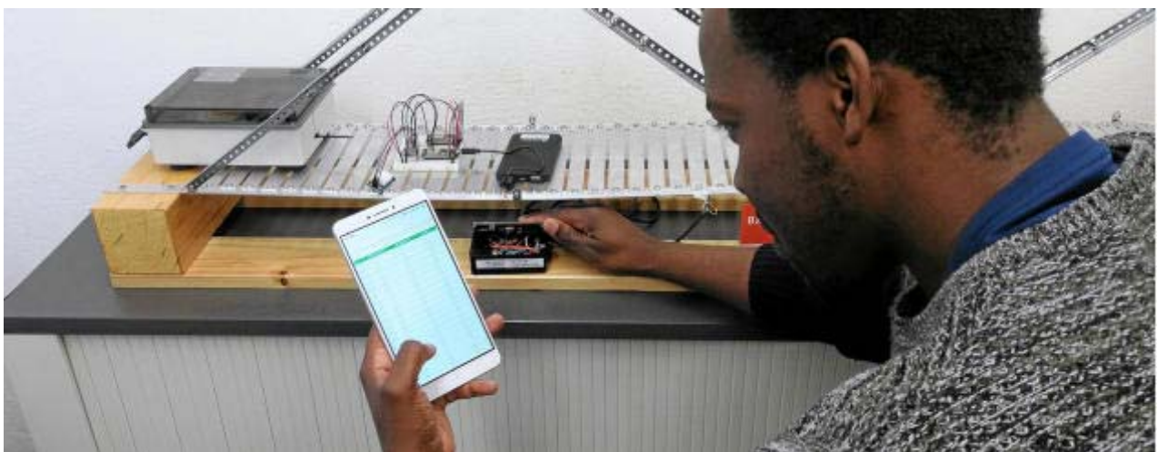
Sensoriklabor Weimar: Everett Mthunzi an einem Modell zur Brückenüberwachung. Foto: Dana Höftmann
