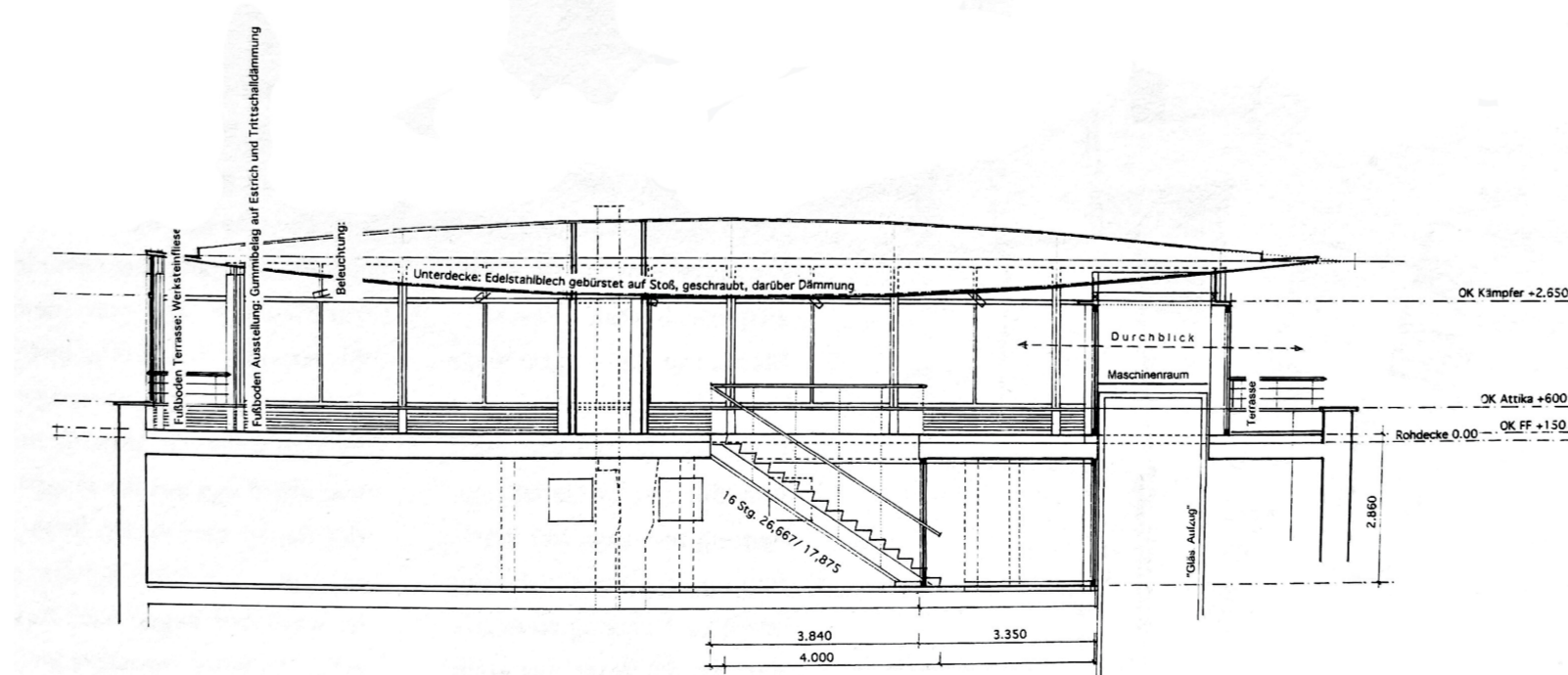
LIMONA-PAVILLON WEIMAR 1994 Entwurfsverfasser: Bernd Rudolf / Torsten Brecht Ingenieurbüro: BGS / Matthias Münz
