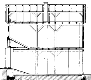
Querschnitt a.
