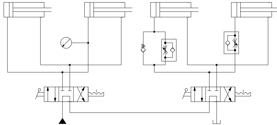
Abbildung 6.1: Eine Beispielschaltung
