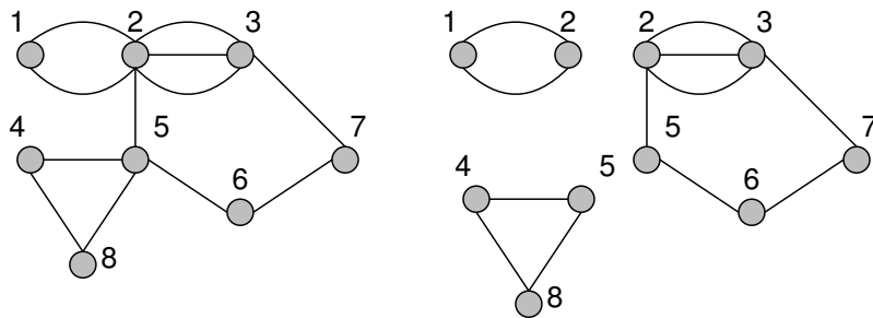
Abbildung 1.5: Ein Graph und seine Blöcke
