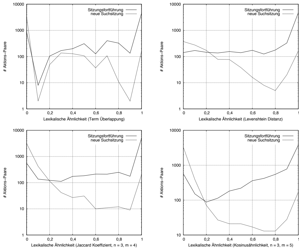
Abbildung 3.7: Ähnlichkeits-Verteilungen der verschiedenen lexikalischen Merkmale
