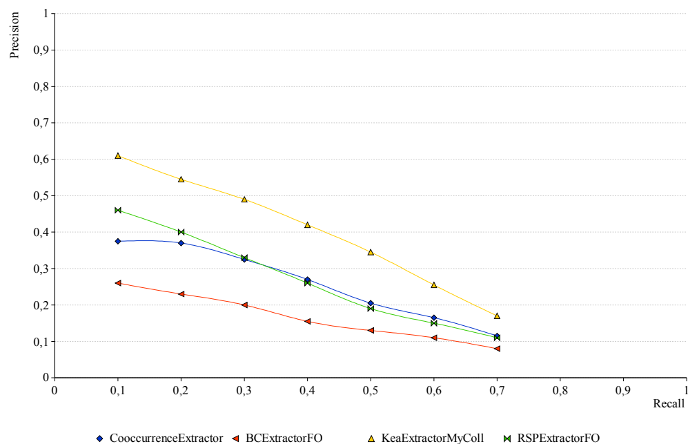
Abbildung 26: Precision-Recall-Kurve
