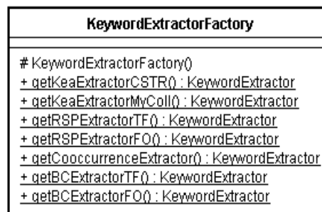
Abbildung 10: Klassendiagramm KeywordExtractorFactory
