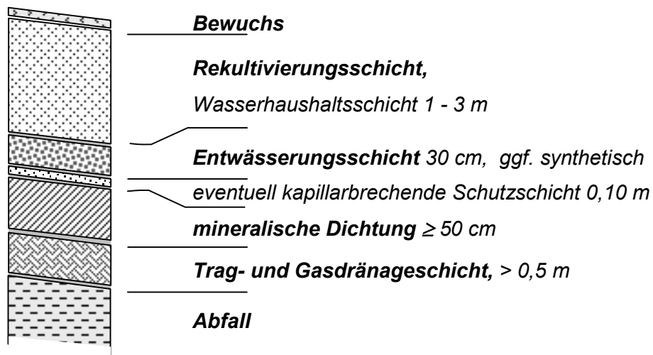
Bild 1: Prinzipschnitt zum Systemaufbau einer mineralischen Oberflächenabdichtung
