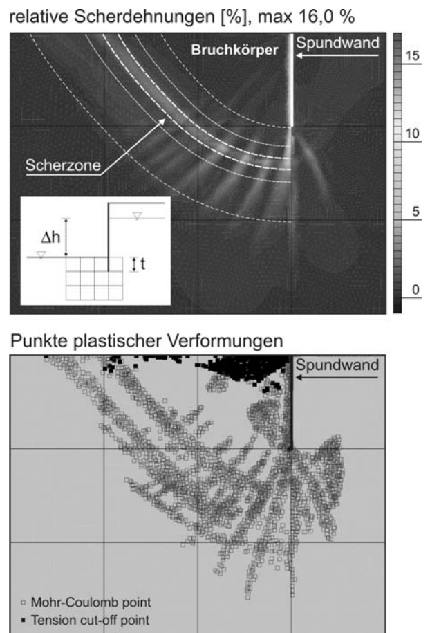
Abbildung 6: Bruchkörperanalyse bei hydraulischer Belastung des baugrubenseitigen Widerlagers; Kohäsion c = 5 kN/m 2
